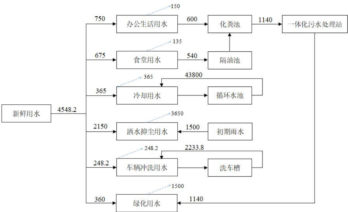
图2-1 水平衡图（单位：m³/a）
