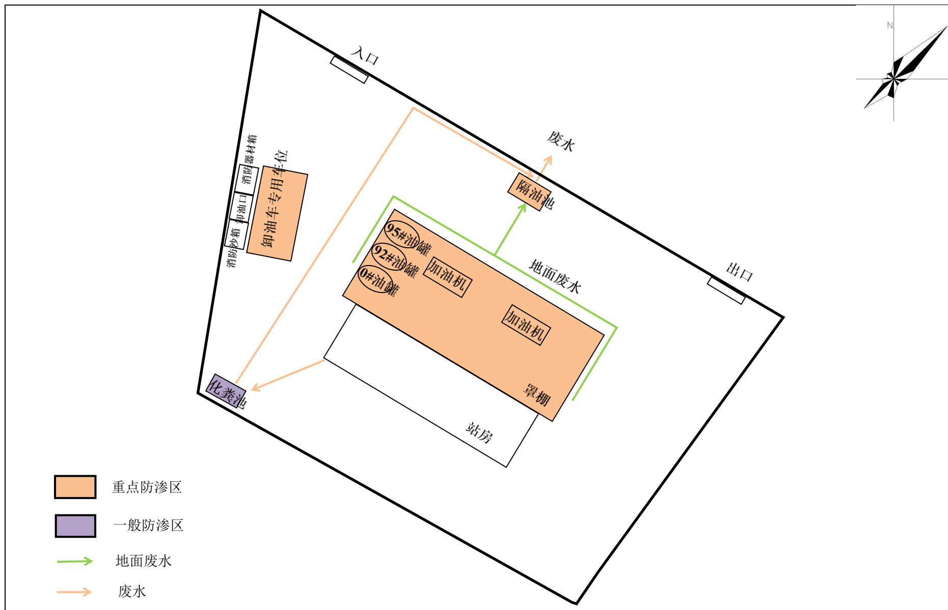
附图3 项目平面布置及雨污管网图
